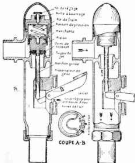
Coupe transversale
