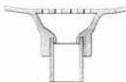
Coupe du départ direct et du tube fer fileté N° 401 - 404 - 422
