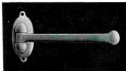
Porte-Serviettes, modèle mobile N° 11, à une branche. Longueur : 40 5 / m Poids approximatif : 900 gr.
