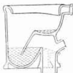
Fig. 565 (coupe)
